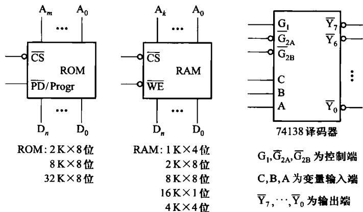
图 4.15 第 36 题芯片图
