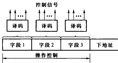
图 10.8 字段直接编码方式
