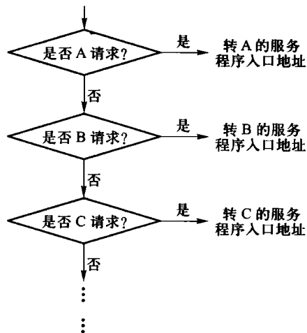
图 8.13 按 A>B>C\cdots 优先级别的软件排队
