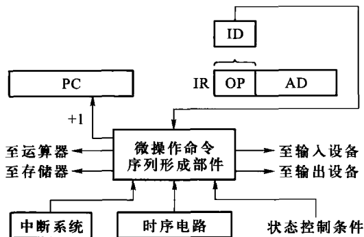
图 10.23 组合逻辑控制器框图
