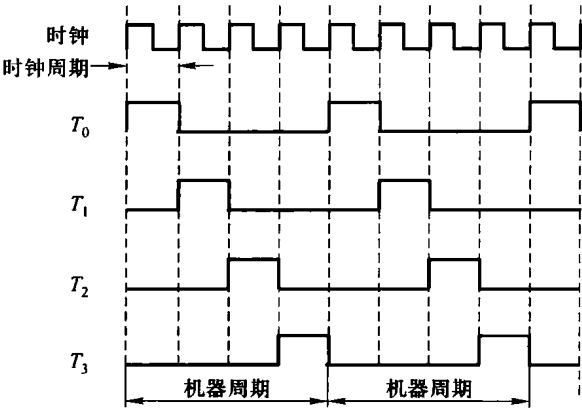
图 9.2 机器周期、时钟周期和节拍的关系
